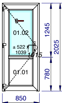
1/50 - Vue intérieure Localisation: Rue des Blancs Chevaux 9/209 à 216 Commun
