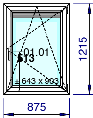
1/50 - Vue intérieure Localisation: Rue des Blancs Chevaux 15/117
