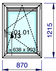
1/50 - Vue intérieure Localisation: Rue des Blancs Chevaux 9/115
