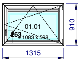
1/50 - Vue intérieure Localisation: Rue des Blancs Chevaux 15/105
