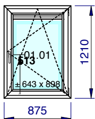
1/50 - Vue intérieure Localisation: Rue des Blancs Chevaux 9/215
