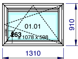
1/50 - Vue intérieure Localisation: Rue des Blancs Chevaux 9/116
