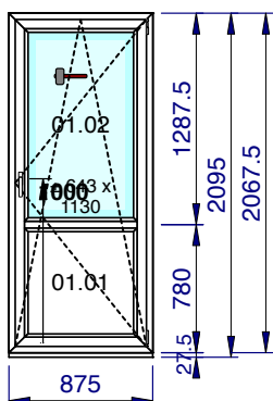
1/50 - Vue intérieure Localisation: Rue des Blancs Chevaux 15/103 à 110 Commun
