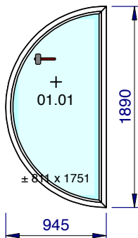
1/50 - Vue intérieure Localisation: Rue des Blancs Chevaux 9/002 06/05/18 - 07:06:07 - WinPro 9.1.0
