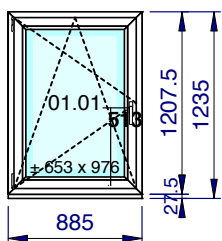
1/50 - Vue intérieure Localisation: Rue des Blancs Chevaux 9/003 à 010 Commun
