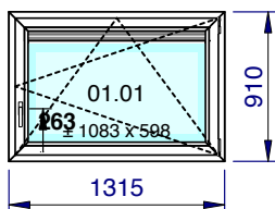
1/50 - Vue intérieure Localisation: Rue des Blancs Chevaux 9/214
