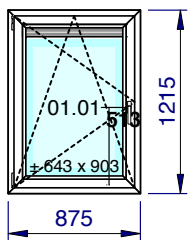
1/50 - Vue intérieure Localisation: Rue des Blancs Chevaux 9/216
