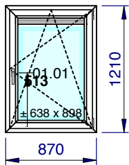
1/50 - Vue intérieure Localisation: Rue des Blancs Chevaux 9/208
