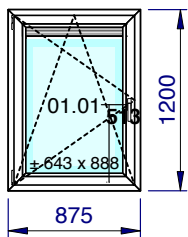
1/50 - Vue intérieure Localisation: Rue des Blancs Chevaux 15/118
