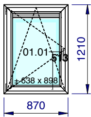
1/50 - Vue intérieure Localisation: Rue des Blancs Chevaux 15/207
