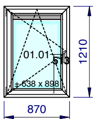
1/50 - Vue intérieure Localisation: Rue des Blancs Chevaux 9/118
