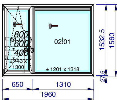
1/50 - Vue intérieure Localisation: Rue des Blancs Chevaux 15/202 Studio
