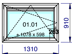
1/50 - Vue intérieure Localisation: Rue des Blancs Chevaux 9/211
