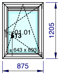
1/50 - Vue intérieure Localisation: Rue des Blancs Chevaux 9/111
