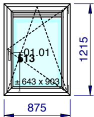
1/50 - Vue intérieure Localisation: Rue des Blancs Chevaux 15/104
