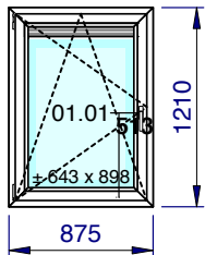
1/50 - Vue intérieure Localisation: Rue des Blancs Chevaux 15/103
