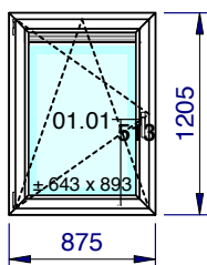
1/50 - Vue intérieure Localisation: Rue des Blancs Chevaux 15/114
