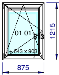
1/50 - Vue intérieure Localisation: Rue des Blancs Chevaux 9/114
