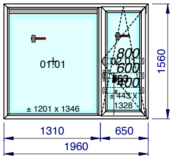
1/50 - Vue intérieure Localisation: Rue des Blancs Chevaux 15/201
