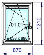
1/50 - Vue intérieure Localisation: Rue des Blancs Chevaux 9/210
